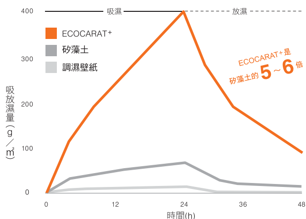
ECOCARAT + 與其它壁材吸放濕量比較
